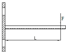
Nosník s nástěnnou konzolou 27×18×1,25
