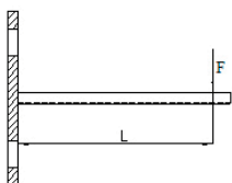
Konzola ST 41×62×3,00
